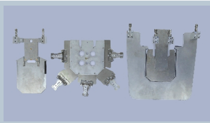
柔性夹具 (选配) Flexible jigs(optional)
